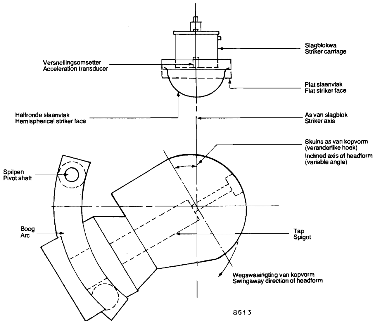
Fig. 4—Skokbreektoetsapparaat Fig. 4—Shock Absorption Test Apparatus
