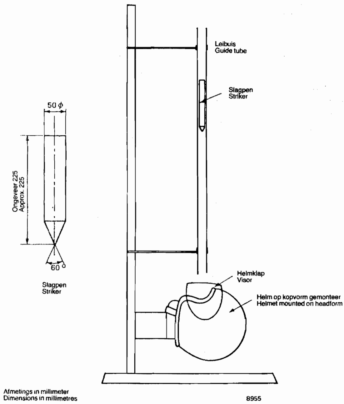
Fig. 8—Toetsapparaat vir Sterkte van Helmklap Fig. 8—Test Apparatus for Visor Strength
