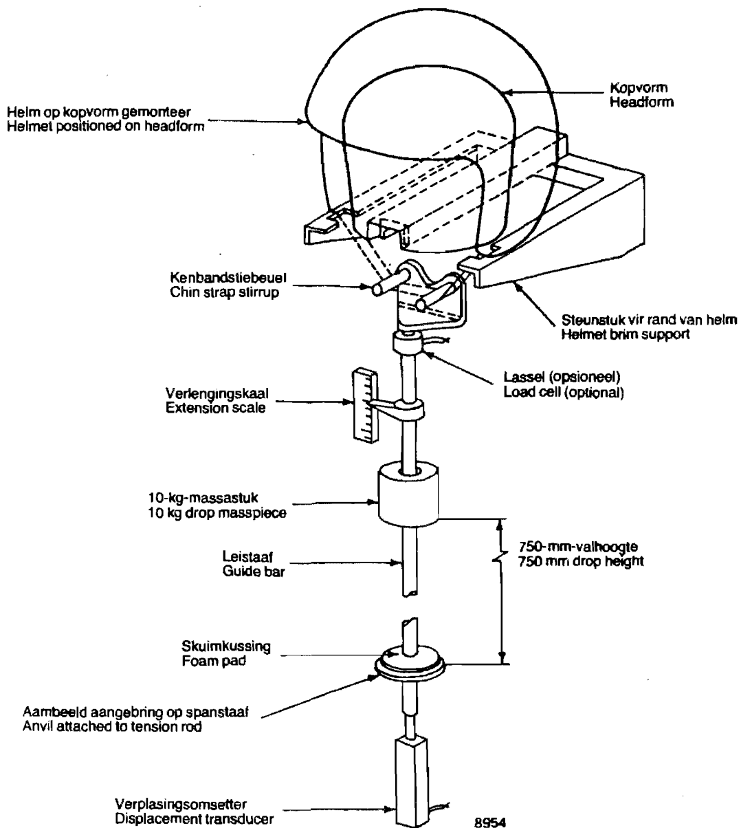
Fig. 6—Toetsapparaat vir Sterkte van Vashousteisel Fig. 6—Retention System Test Apparatus
