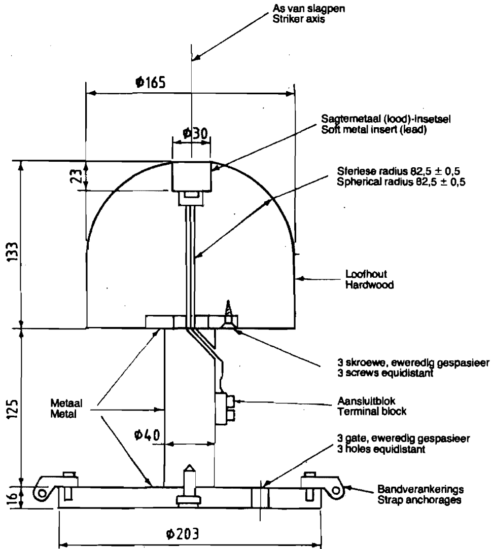
Afmetings in millimeter behoudens 'n toleransie van \pm 1 mm Dimensions in millimetres tolerance \pm 1 mm
